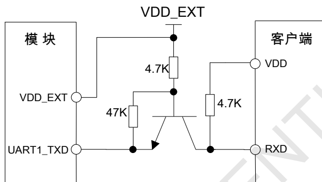
图 13: TXD 连接图
