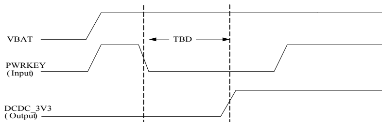
图 20: VDD_3V3 上电时序图
