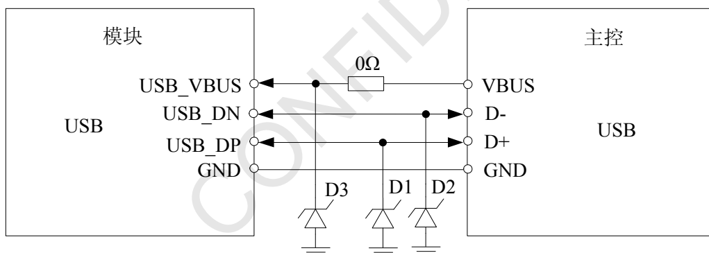
图 16: USB 连接图
