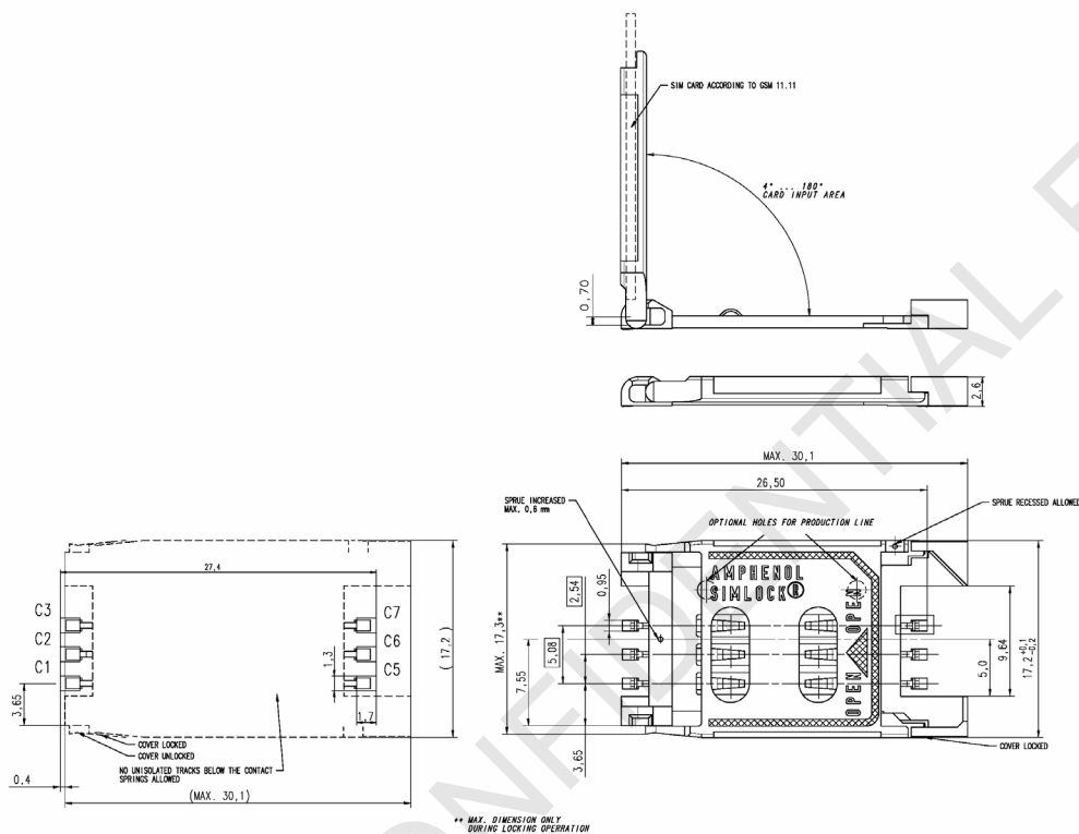
图 18: Amphenol C707 10M006 512 SIM 卡座尺寸图
