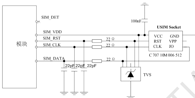
图 17: SIM 接口推荐电路
