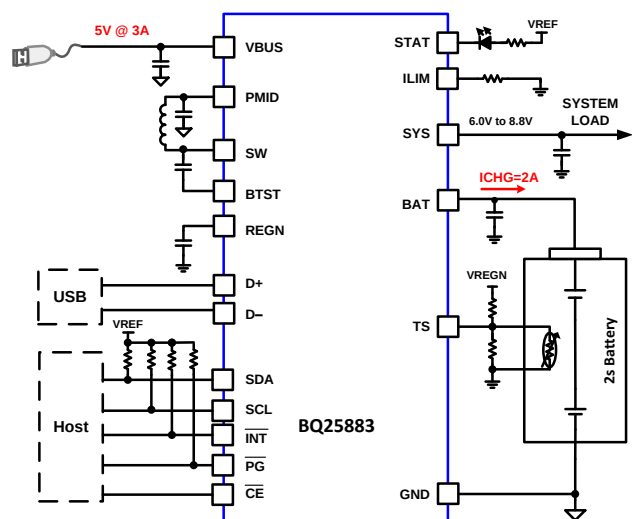
简化原理图
