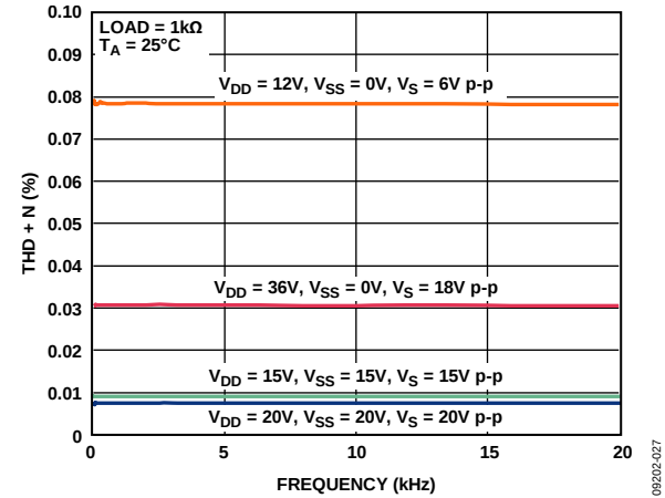
图20. THD + N与频率的关系( \pm 15 V双电源)
