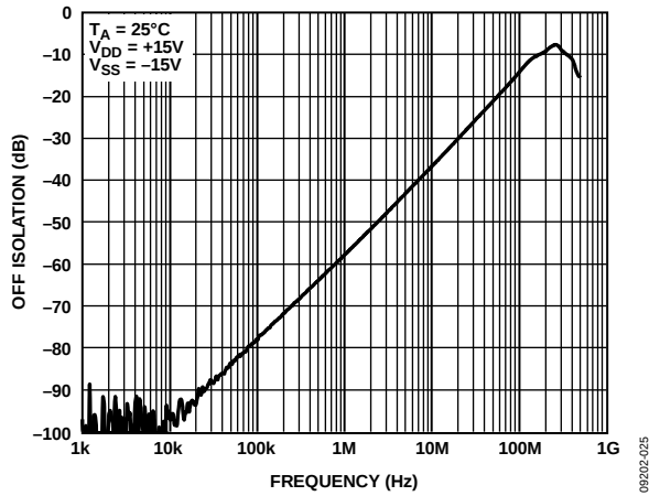
图16. 关断隔离与频率的关系( \pm 15 V双电源)
