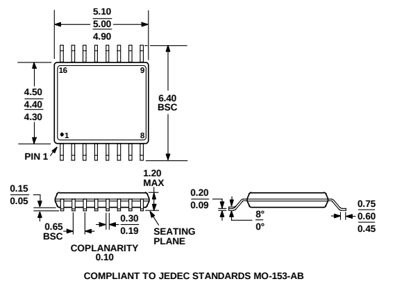
图34. 16引脚，超薄紧缩小型封装[TSSOP] (RU-16) 图示尺寸单位：毫米
