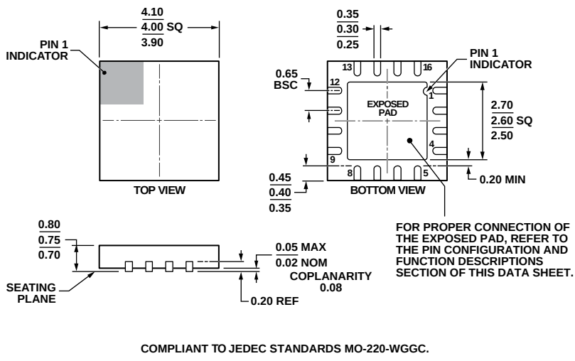
图35. 16引脚，引脚架构芯片级封装[LFCSP_WQ] 4 mm×4 mm，超薄体 (CP-16-17) 图示尺寸单位：毫米
