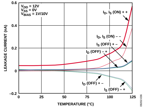
图14. 漏电流与温度的关系(12 V单电源)
