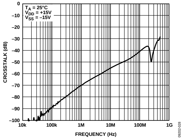
图17. 串扰与频率的关系( \pm 15 V双电源)
