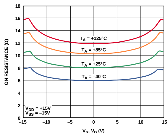
图8. 不同温度下 R_{ON} 与 V_S (V_D) 的关系 ( \pm 15\text{V} 双电源)
