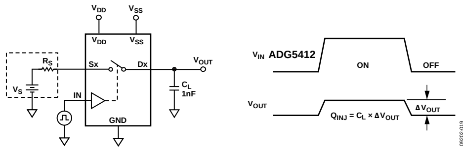
图32. 电荷注入
