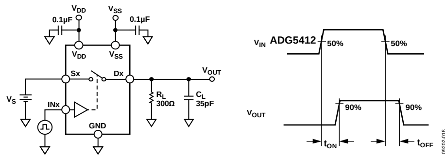
图31. 开关时间
