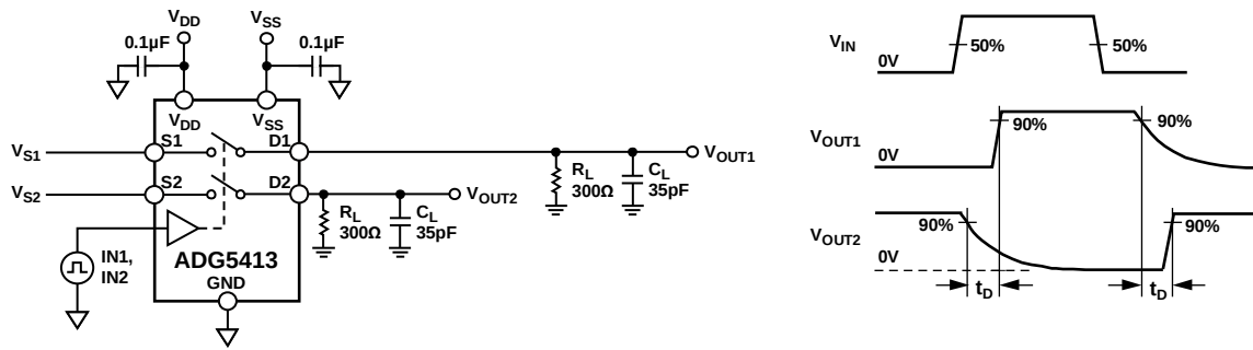
图30. 先开后合时间延迟 t_D
