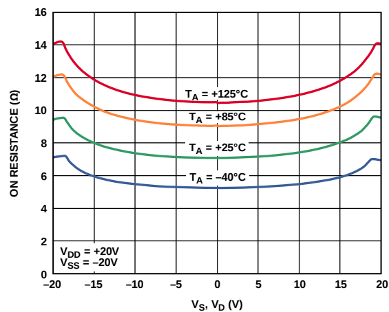
图9. 不同温度下 R_{ON} 与 V_S (V_D) 的关系 ( \pm 20\text{V} 双电源)
