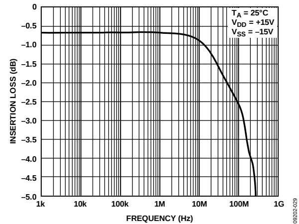
图21. 带宽
