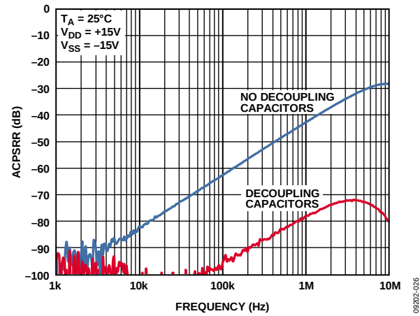
图19. ACPSRR与频率的关系( \pm 15 V双电源)
