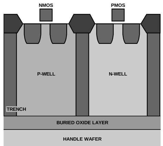
图33. 沟槽隔离
