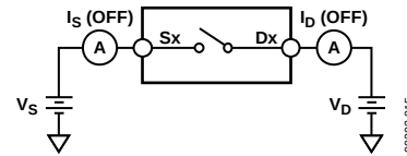
图27. 关断泄漏
