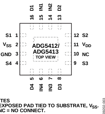
图3. LFCSP引脚配置
