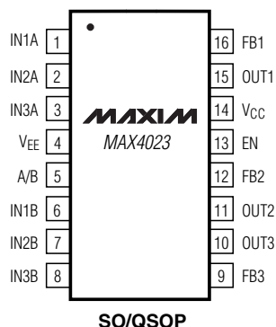
SO/QSOP
