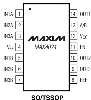
SO/TSSOP
