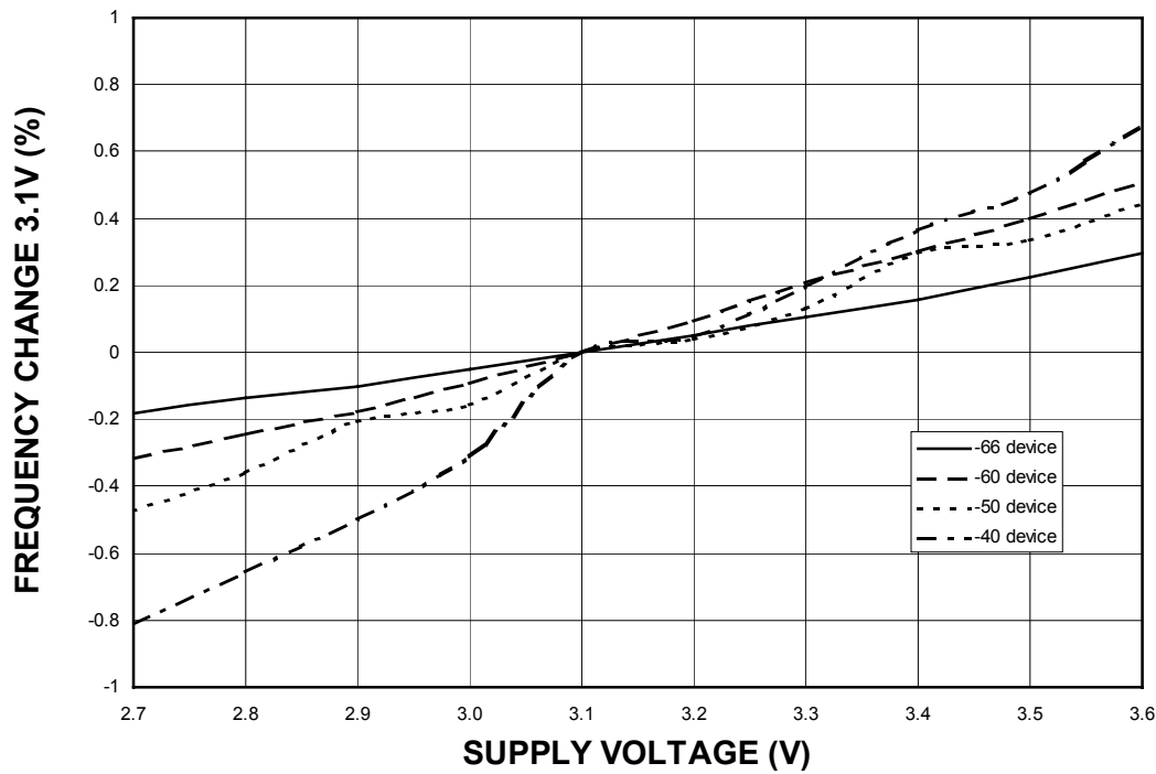
DS1077L VOLTCO
