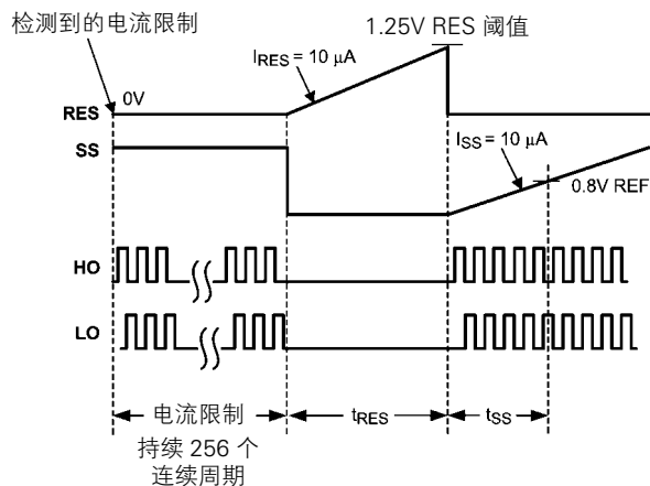
图 11: 打嗝模式电流限制时序图
