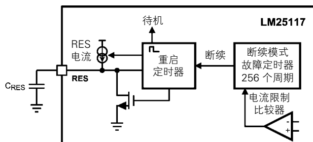
图 12: 打嗝模式电流限流电路
