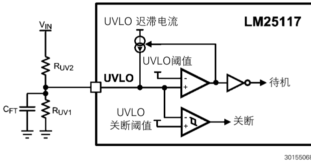
图 6: UVLO 配置
