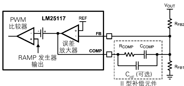
图 9：反馈配置和 PWM 比较器
