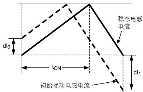
图 16: dl_1/dl_0 < -1 时的初始扰动效应
