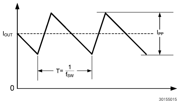
图 10: 电感电流
