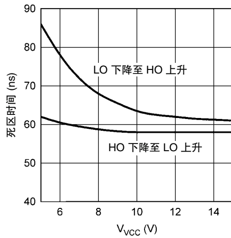
驱动器死区时间与 V_{CC} 的关系
