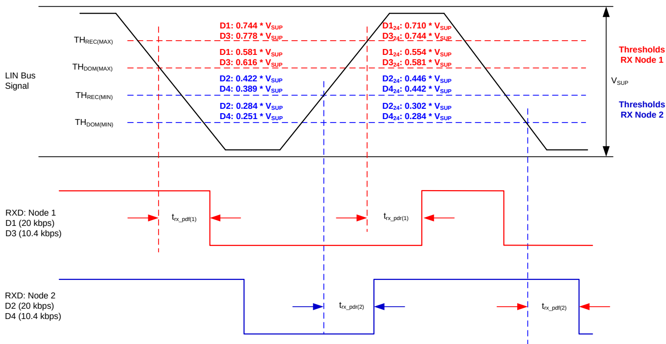
图 21. Propagation Delay
