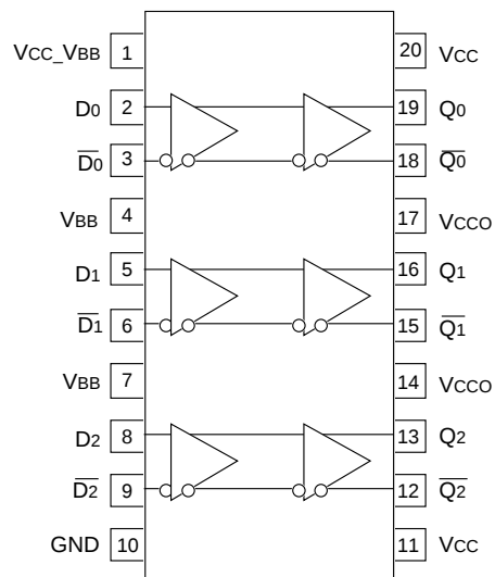
20-Pin Wide SOIC (Z20-1)
