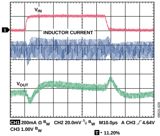
图29. 线路瞬态响应, V_{OUT} = 1.8\text{ V} , PWM模式, 800 mA, V_{INI} = 4\text{ V} 至 5\text{ V} , 2\mu\text{s} 上升时间, C_{IN} = 3.3\mu\text{F}
