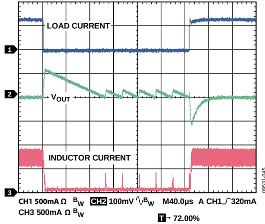
图45. 负载瞬态响应, V_{OUT} = 1.2 V, 10 mA至800 mA, 负载电流上升时间 = 200 ns, V_{IN} = 5 V
