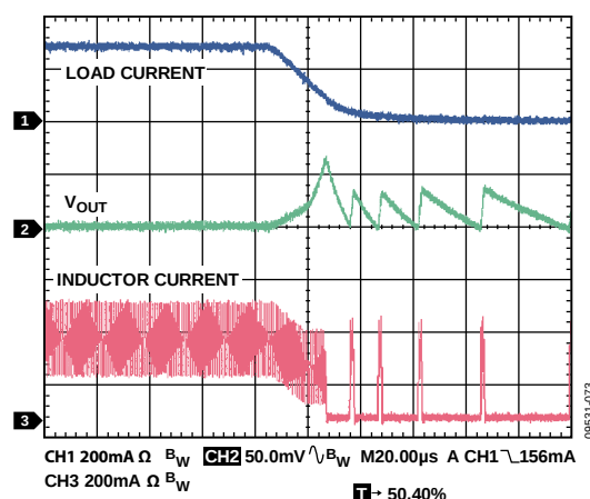
图73. PWM至PSM转换波形， V_{OUT} = 1.8 V ，300 mA至10 mA负载
