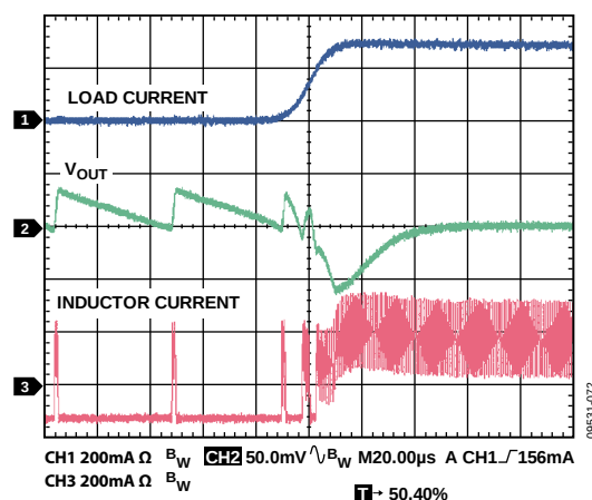
图72. PSM至PWM转换波形， V_{OUT} = 1.8 V ，10 mA至300 mA负载
