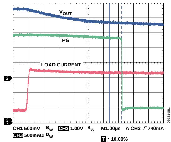
图81. 200 mA至1100 mA负载瞬态下的典型PG时序
