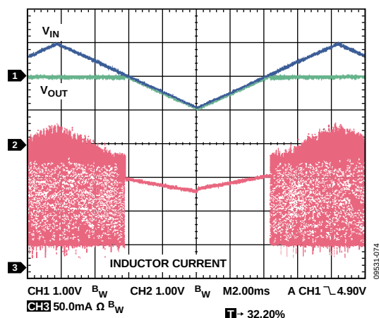
图74. PSM模式下进入和退出100%占空比， V_{OUT} = 5V ，100 mA负载
