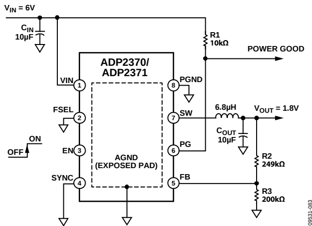
图83. 典型应用，600 kHz，可调输出
