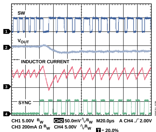
图78. SYNC瞬态响应，1.2 MHz至800 kHz
