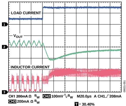
图51. 负载瞬态响应, V_{OUT} = 5\text{ V} , 100 mA至300 mA, 负载电流上升时间 = 200 ns, V_{IN} = 8\text{ V}
