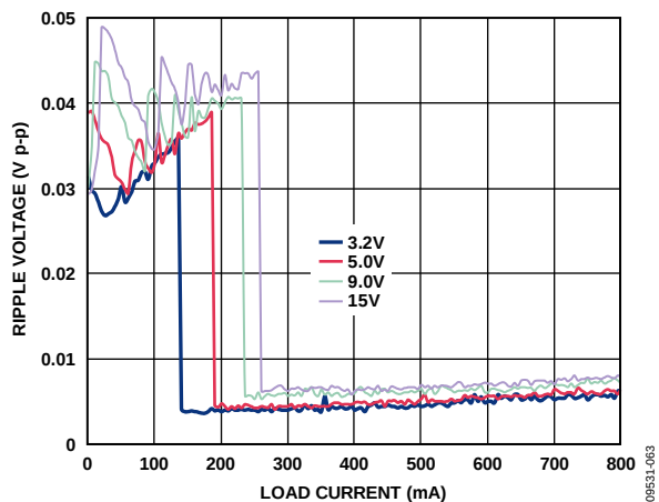
图63. 不同输入电压下输出纹波与负载电流的关系, V_{OUT} = 1.8\text{ V} , 自动模式
