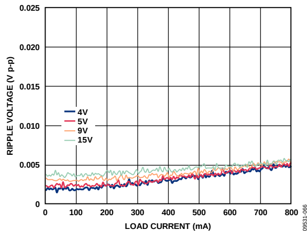
图66. 不同输入电压下输出纹波与负载电流的关系, V_{OUT} = 3.3\text{ V} , 强制PWM模式
