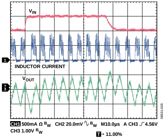
图28. 线路瞬态响应, V_{OUT} = 1.8\text{ V} , PSM模式, 100 mA, V_{INI} = 4\text{ V} 至 5\text{ V} , 2\mu\text{s} 上升时间, C_{IN} = 3.3\mu\text{F}
