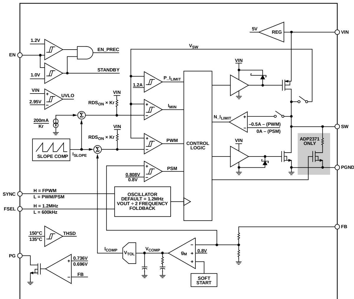
图71. 功能框图
