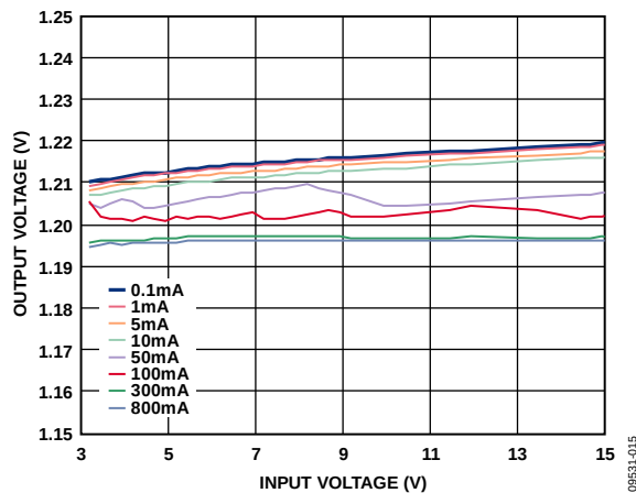
图15. 不同负载下的电压调整率, V_{OUT} = 1.2V
