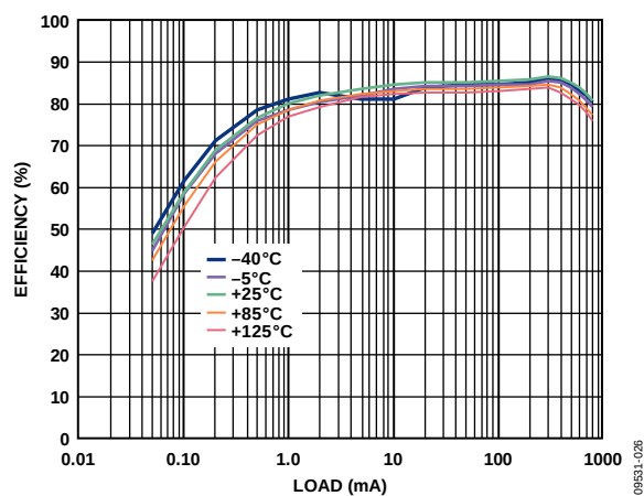
图26. 不同温度下效率与负载电流的关系, V_{OUT} = 1.8V , V_{IN} = 4V
