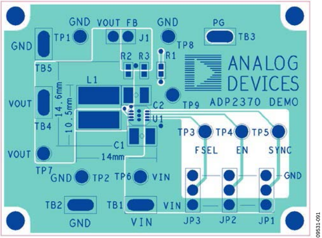
图91. PCB布局布线(顶部)
