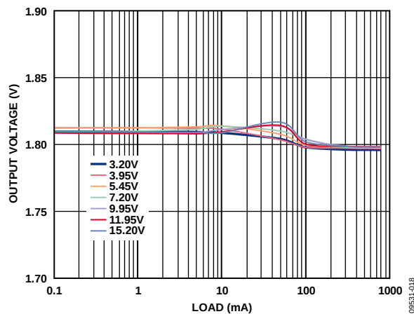
图18. 负载调整率, V_{OUT} = 1.8V
