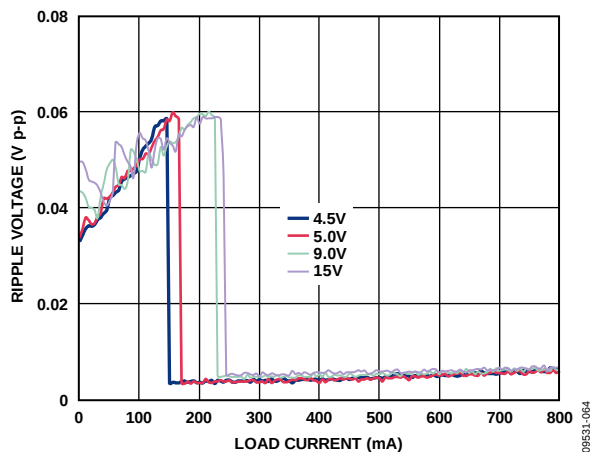
图64. 不同输入电压下输出纹波与负载电流的关系, V_{OUT} = 3.3\text{ V} , 自动模式
