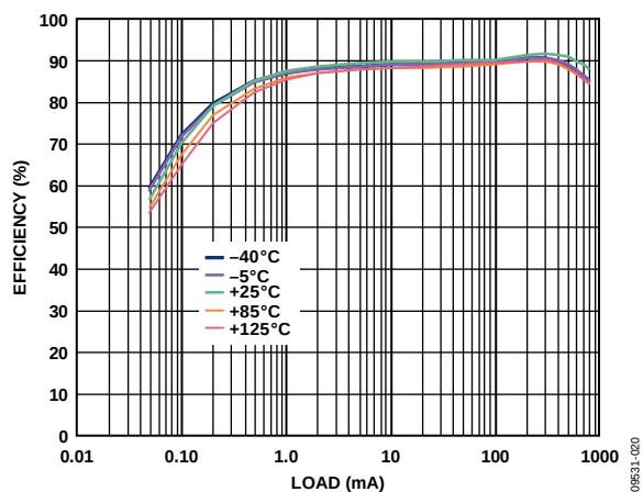
图20. 不同温度下效率与负载电流的关系, V_{OUT} = 3.3V , V_{IN} = 7.3V
