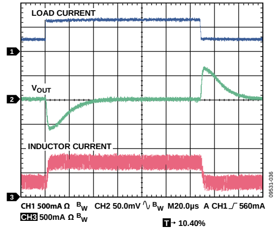
图36. 负载瞬态响应, V_{OUT} = 1.8 V, 300 mA至800 mA, 负载电流上升时间 = 200 ns
