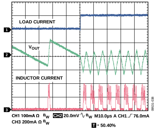
图38. 负载瞬态响应, V_{OUT} = 1.8 V, 10 mA至110 mA, 负载电流上升时间 = 200 ns
