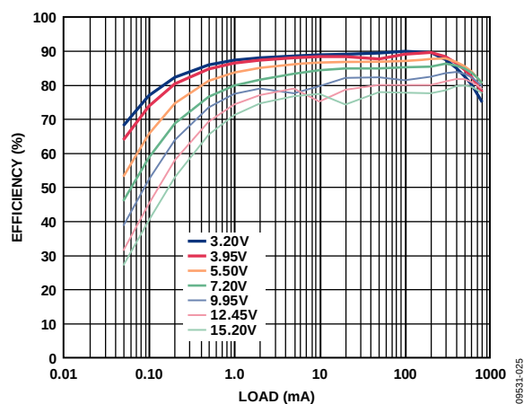
图25. 不同输入电压下效率与负载电流的关系, V_{OUT} = 1.8V
