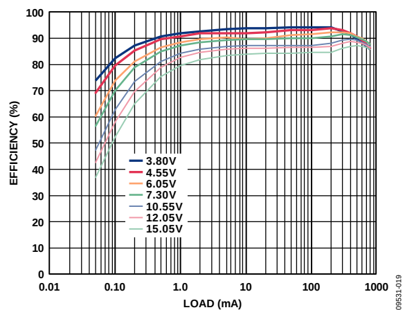
图19. 不同输入电压下效率与负载电流的关系, V_{OUT} = 3.3V
