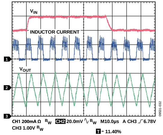
图32. 线路瞬态响应, V_{OUT} = 3.3\text{ V} , PSM模式, 100 mA, V_{INI} = 6\text{ V} 至 7\text{ V} , 2\mu\text{s} 上升时间, C_{IN} = 3.3\mu\text{F}
