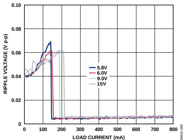
图65. 不同输入电压下输出纹波与负载电流的关系, V_{OUT} = 5\text{ V} , 自动模式
