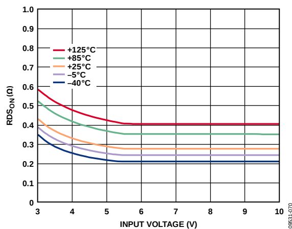
图70. 不同温度下NMOS R_{DS_{ON}} 与输入电压的关系, 400 mA
