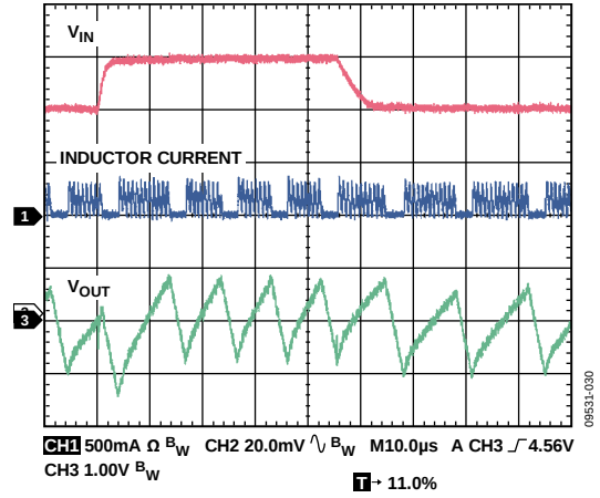
图30. 线路瞬态响应, V_{OUT} = 1.2\text{ V} , PSM模式, 100 mA, V_{INI} = 4\text{ V} 至 5\text{ V} , 2\mu\text{s} 上升时间, C_{IN} = 3.3\mu\text{F}
