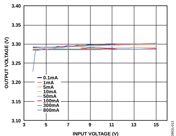
图13. 不同负载下的电压调整率, V_{OUT} = 5.0\text{ V}
