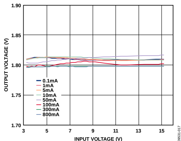
图17. 不同负载下的电压调整率, V_{OUT} = 1.8V
