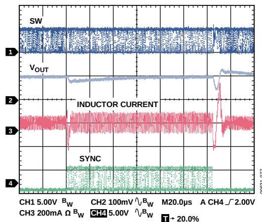
图77. SYNC典型瞬态响应，1.2 MHz至800 kHz至1.2 MHz
