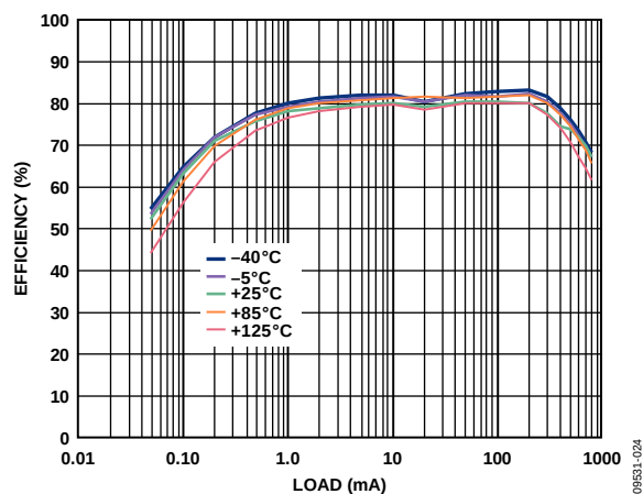
图24. 不同温度下效率与负载电流的关系, V_{OUT} = 1.2V , V_{IN} = 4V
