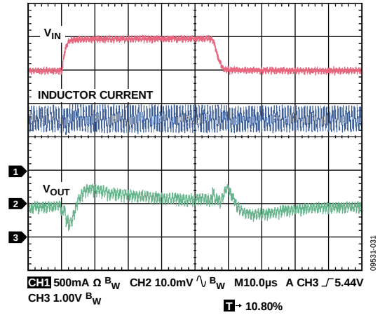
图31. 线路瞬态响应, V_{OUT} = 1.2\text{ V} , PWM模式, 800 mA, V_{INI} = 4\text{ V} 至 5\text{ V} , 2\mu\text{s} 上升时间, C_{IN} = 3.3\mu\text{F}
