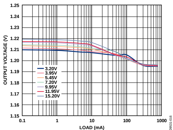
图16. 负载调整率, V_{OUT} = 1.2V
