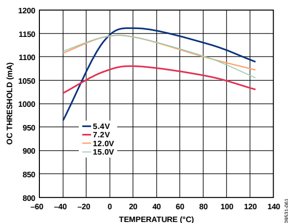
图61. 不同输入电压下过流限值与温度的关系, V_{OUT} = 5V
