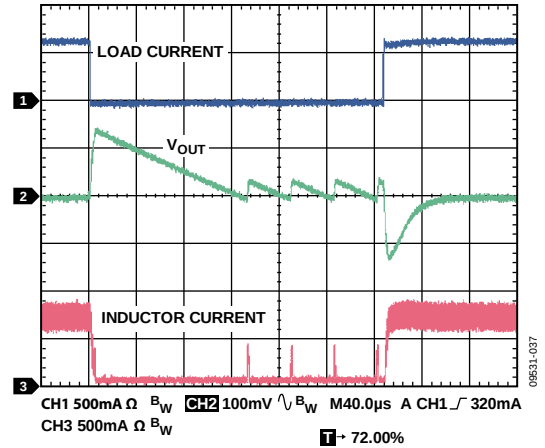
图37. 负载瞬态响应, V_{OUT} = 1.8 V, 10 mA至800 mA, 负载电流上升时间 = 200 ns
