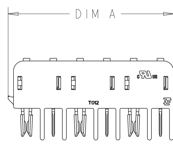
2213288-3/ 1-2213288-3 SCALE 3:1
