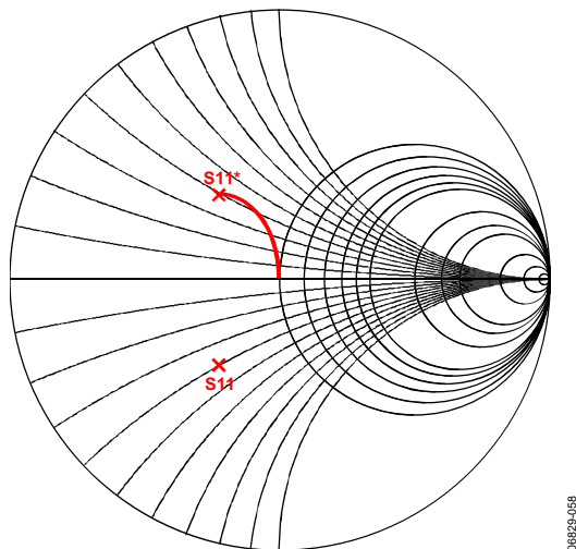
图60. 共轭匹配的史密斯图表现形式
