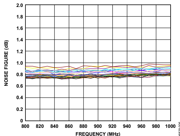
图6. 噪声系数与频率的关系(25°C, 多器件)
