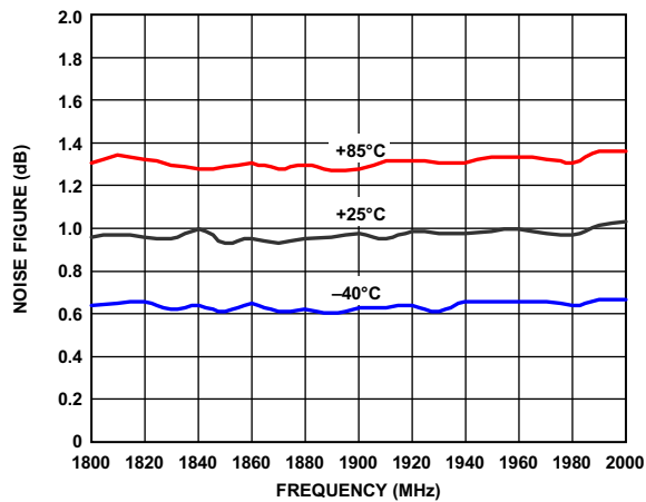
图35. 噪声系数与温度的关系
