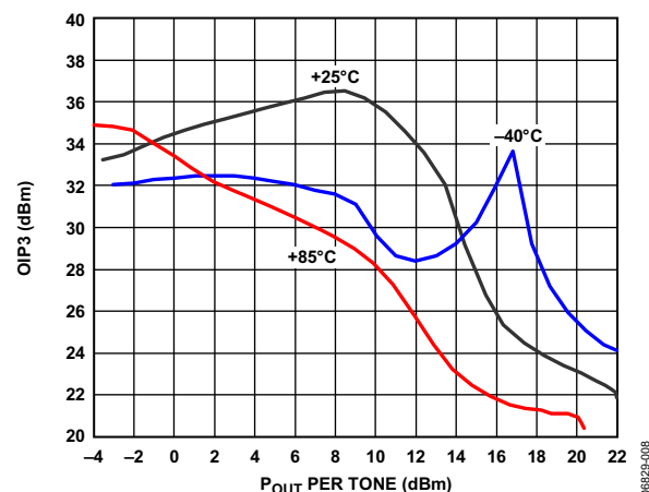
图8. OIP3与输出功率( P_{OUT} )和温度的关系
