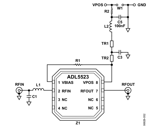
图53. ADL5523基本连接
