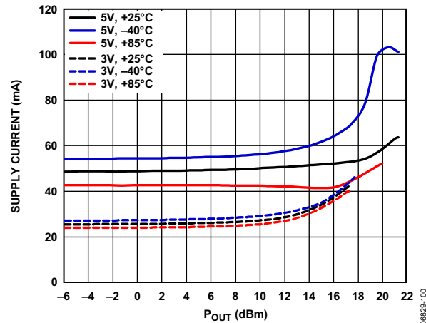
图52. 电源电流与 P_{OUT} 和温度的关系(3 V和5 V)
