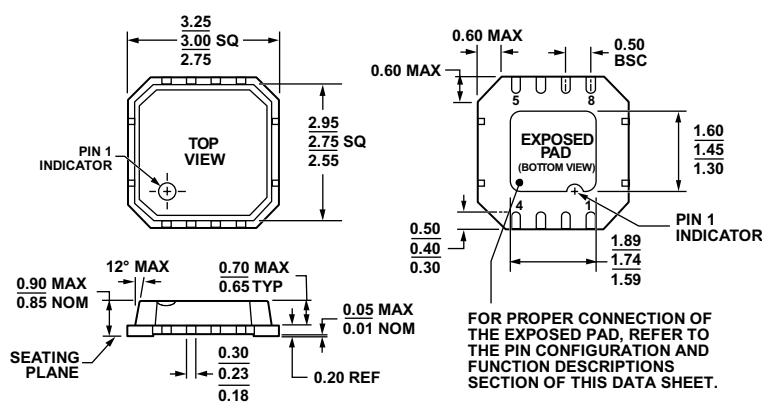
图65. 8引脚脚架构芯片级封装[LFCSP_VD] 3 mm x 3 mm, 超薄体, 双列引脚(CP-8-2) 尺寸单位: mm
