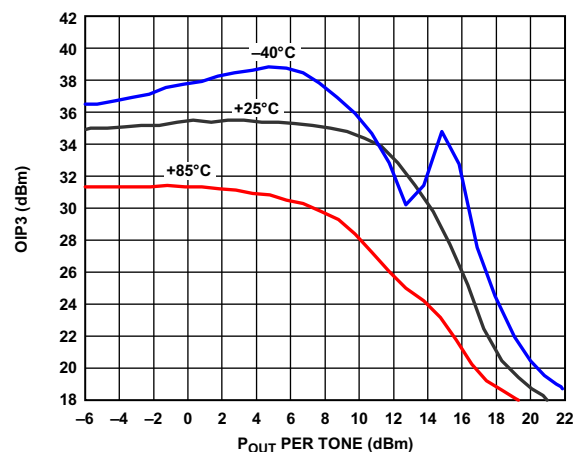
图20. OIP3与输出功率( P_{OUT} )和温度的关系
