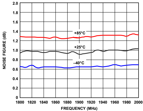
图11. 噪声系数与温度的关系
