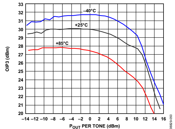
图50. OIP3与输出功率( P_{OUT} )和温度的关系
