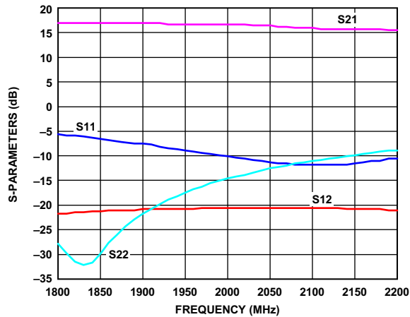
图33. 典型S参数，对数幅度
