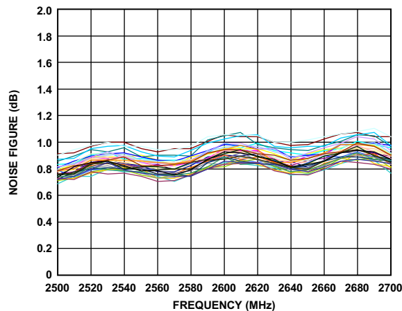
图18. 噪声系数与频率的关系(25°C, 多器件)
