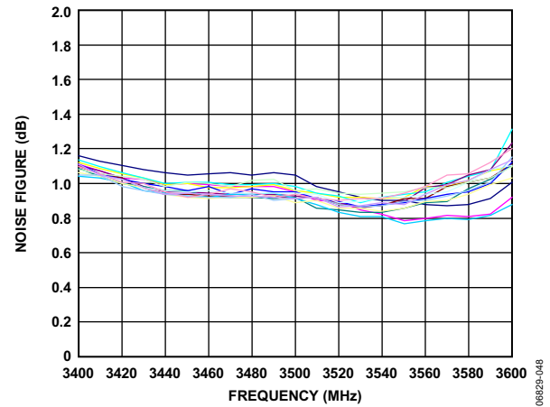
图48. 噪声系数与频率的关系(25°C, 多器件)
