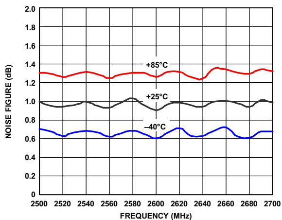
图17. 噪声系数与温度的关系
