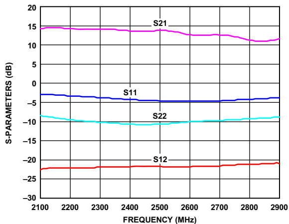
图39. 典型S参数，对数幅度
