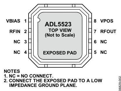
图2. 引脚配置
