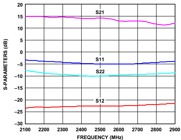
图15. 典型S参数，对数幅度
