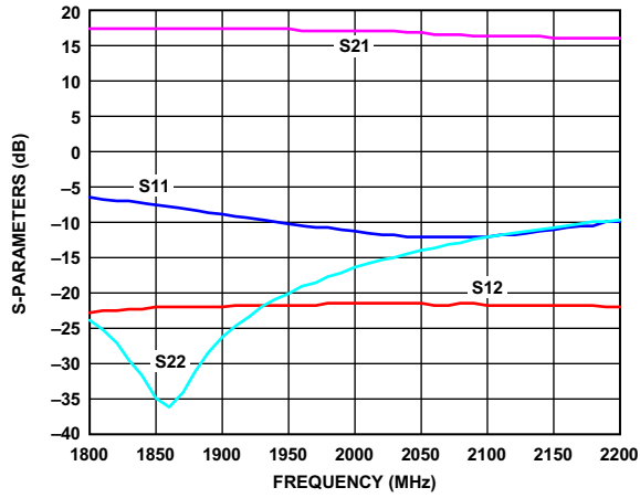
图9. 典型S参数，对数幅度
