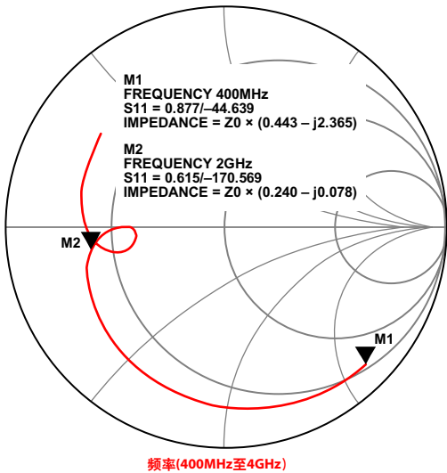
图63. ADL5523的S11(S22为2 GHz匹配)
