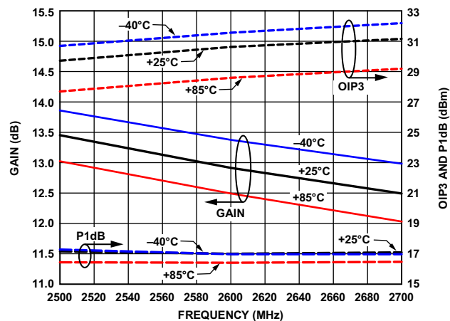
图43. 增益、OIP3和P1dB与温度的关系
