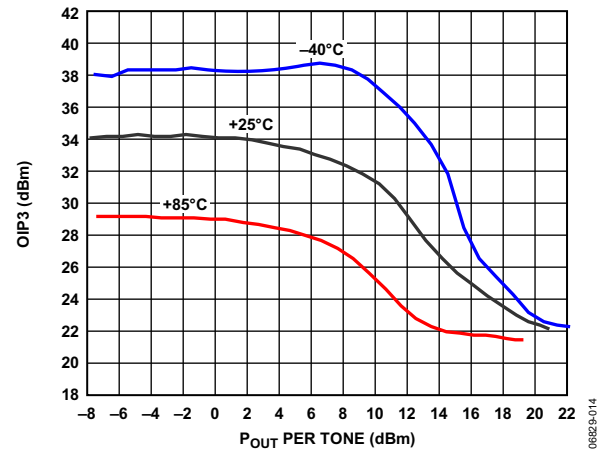
图14. OIP3与输出功率( P_{OUT} )和温度的关系
