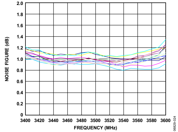
图24. 噪声系数与频率的关系(25°C, 多器件)
