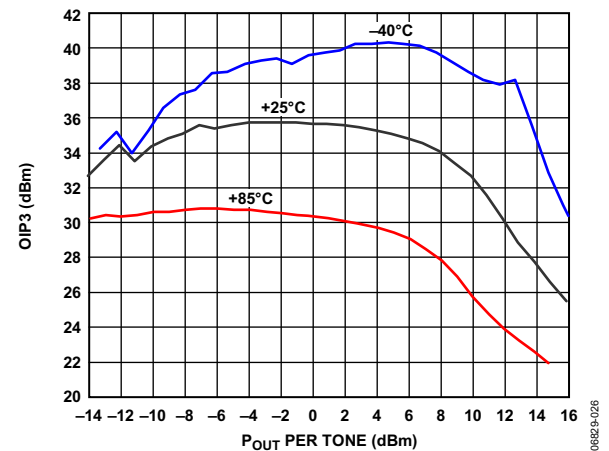
图26. OIP3与输出功率( P_{OUT} )和温度的关系
