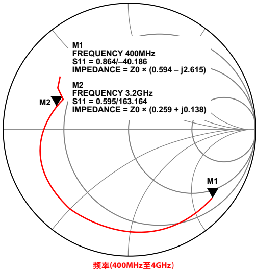
图64. ADL5523的S11(S22为3.2 GHz匹配)
