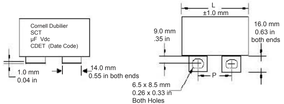
上视图 Top View
