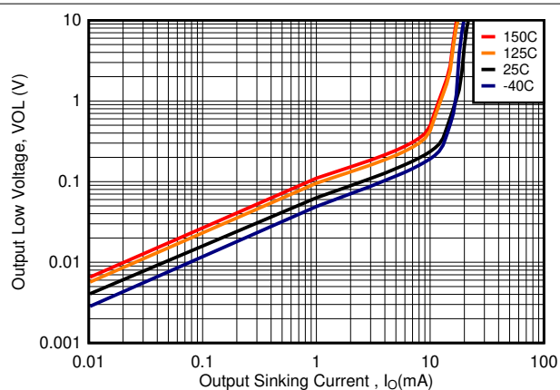
图 3-6. Output Low Voltage vs. Output Current LM2903E-Q1 Only
