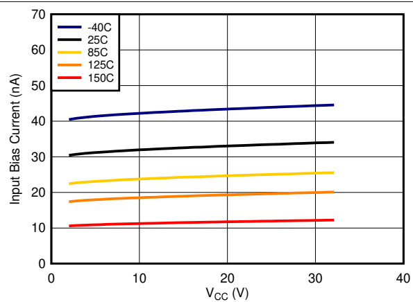
图 3-4. Input Bias Current vs. Supply Voltage LM2903E-Q1 Only
