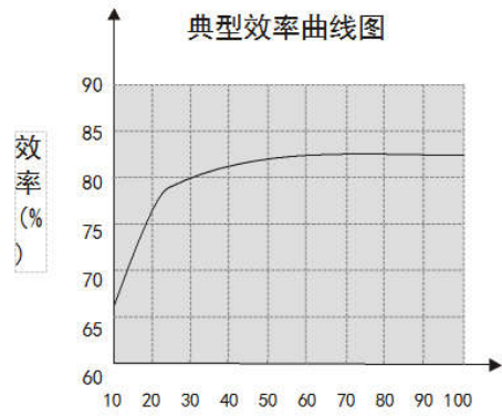
典型效率曲线图
