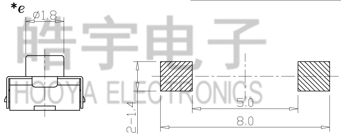
P.C.B LAND DIMENSION
