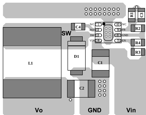
Top Layer
