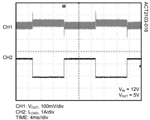
Load Transient (1.5A~3A)
