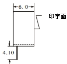
側視圖
