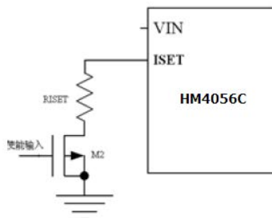
图 5. HM4056C 的使能设计
