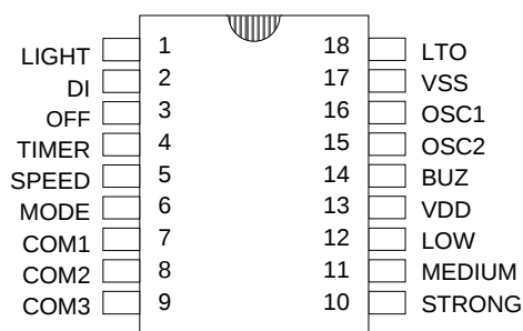
SM3502-A 18PIN
