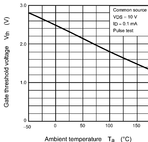
Fig. 7.6 V_{th} - T_a
