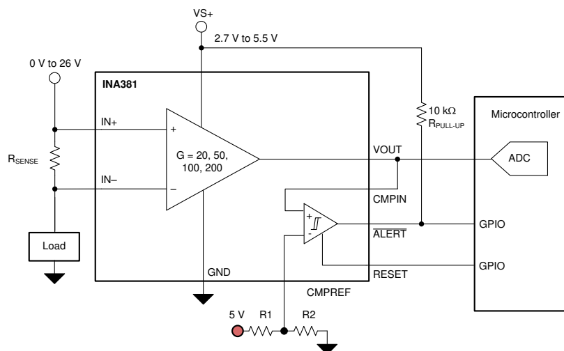
典型应用
