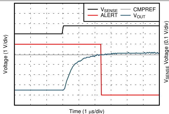
图 32. Brownout Recovery
