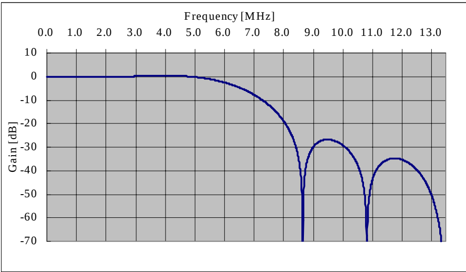
Fig. 3 Chroma-2 LPF
