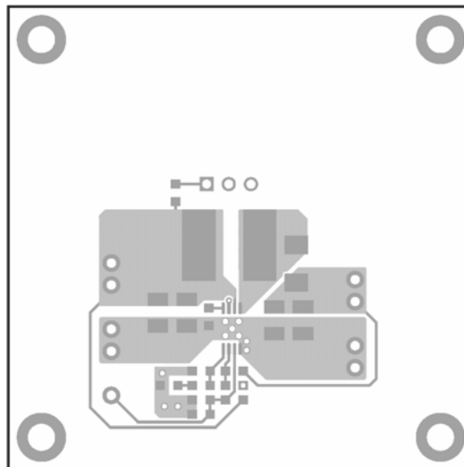
Figure 2—Top Layer
