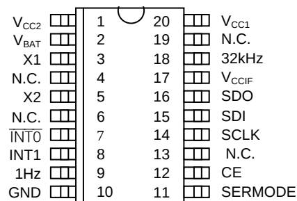
TSSOP (4.4mm)
