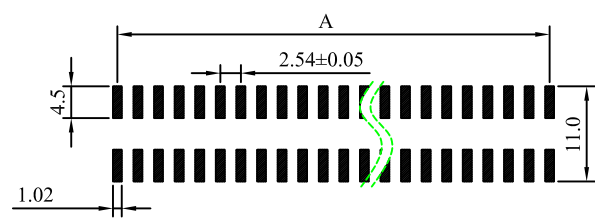
P.C.B Hole Layout
