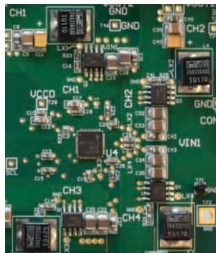
XRP7714EVB
