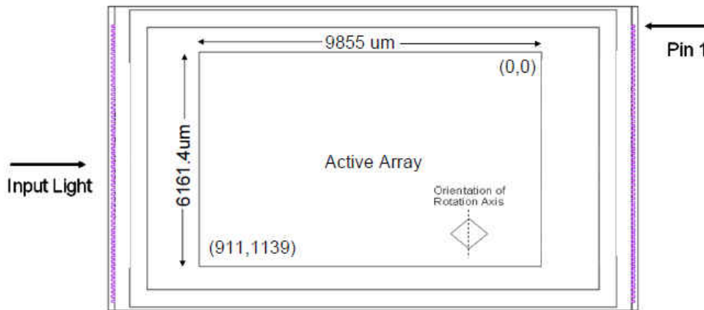
图 7-5. DLP4500 Micromirror Active Area
