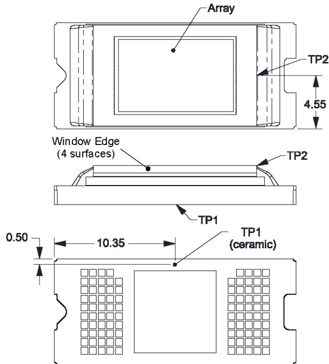
图 8-4. Thermal Test Point Location - FQD Package
