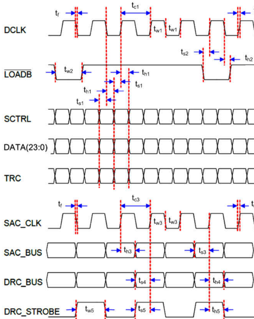
图 7-2. Timing Diagram
