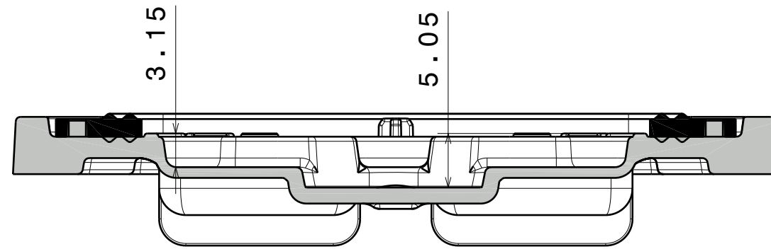
Section view A-A Scale: 2:1
