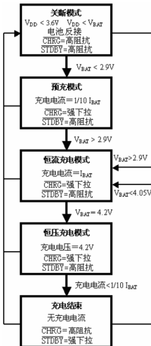
图 1 典型充电循环状态图
