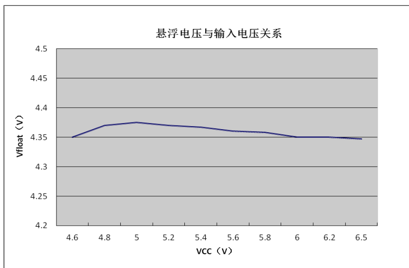
△Figure 12. 悬浮电压与输入电压关系图 (测试条件: BAT 脚接 10uF 电容, RPROG=2.4K)
