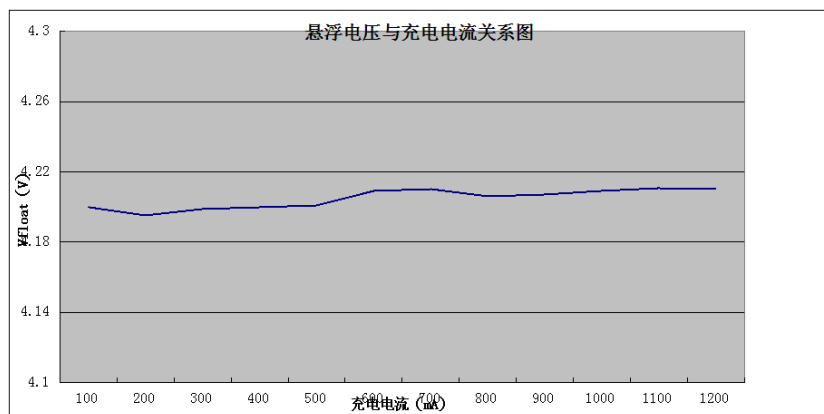
* Figure 8. 悬浮电压与充电电流关系图 (测试条件: VCC=5V)
