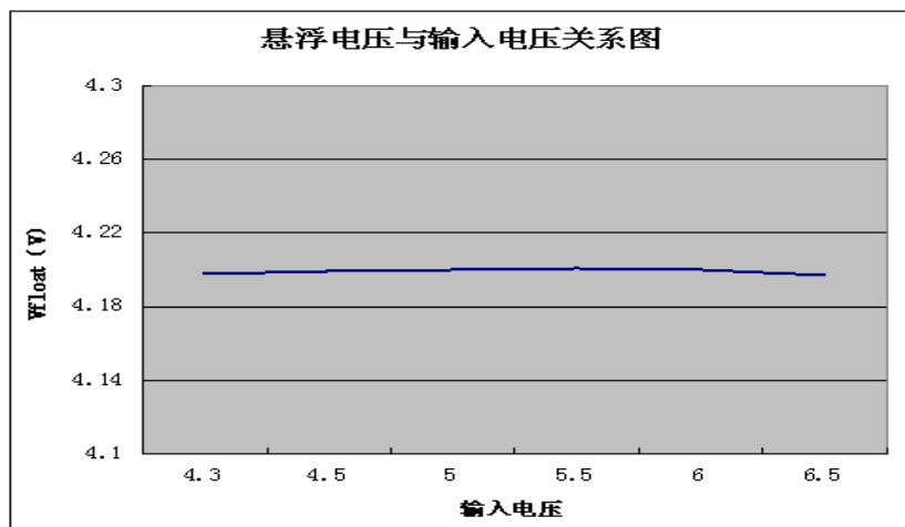
* Figure 4. 悬浮电压与输入电压关系图（测试条件：BAT 脚接 10uF 电容，RPROG=2.4K）
