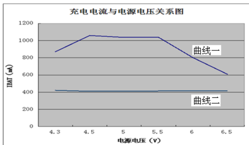
Figure 6. 充电电流与电源电压关系（测试条件：VBAT=4V，曲线一 RPROG=1K，曲线二
