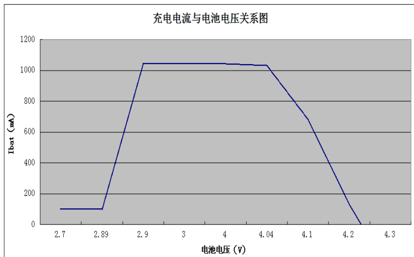
* Figure 9. 充电电流与电池关系图 (测试条件: VCC=5V, Rprog=1.2K)
