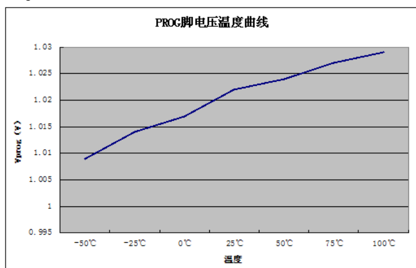
* Figure 2. PROG 脚电压温度曲线 (测试条件: V_{CC}=5\text{V} , V_{\text{BAT}}=3.7\text{V} , R_{\text{PROG}}=2.4\text{K} )
