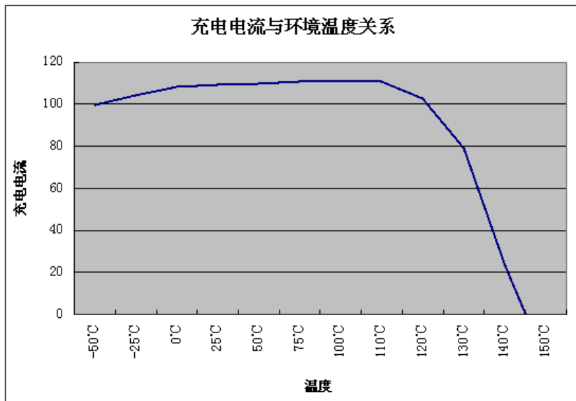
* Figure 7. 充电电流与环境温度关系 (VCC=5V , VBAT=4V, RPOG=10K)
