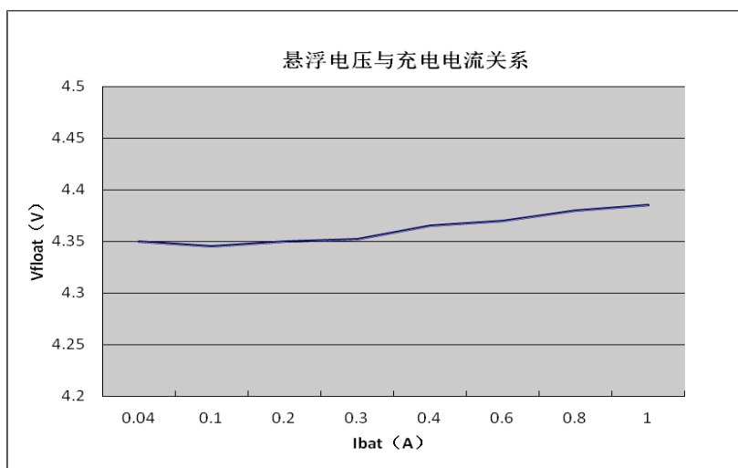
△Figure 14. 悬浮电压与充电电流关系图 (测试条件: VCC=5V)
