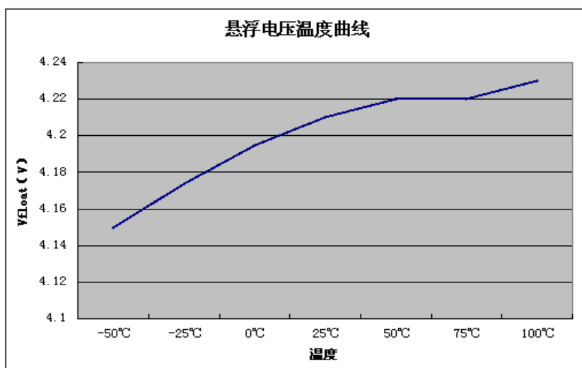
*Figure 1. 悬浮电压曲线图 (测试条件: V_{CC}=5\text{V} , R_{\text{PROG}}=2.4\text{K} )
