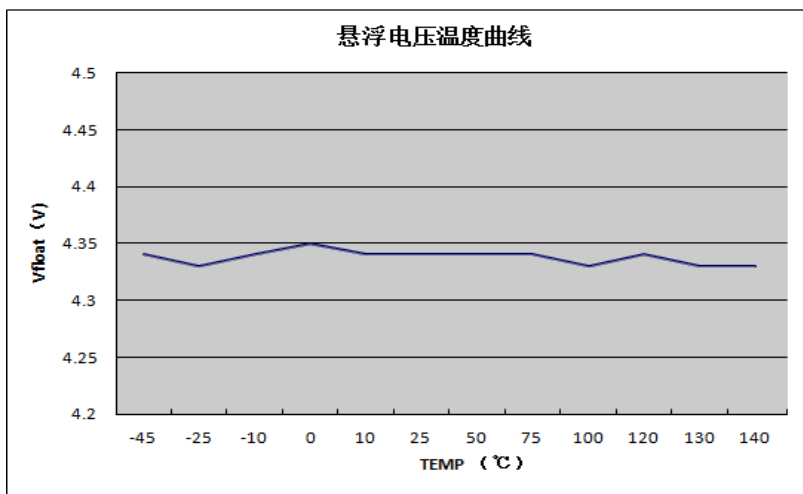
△Figure 10. 悬浮电压温度曲线图 (测试条件: VCC=5V, RPROG=2.4K)
