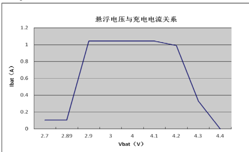
△Figure 15. 充电电流与电池关系图 (测试条件: VCC=5V, Rprog=1.2K)
