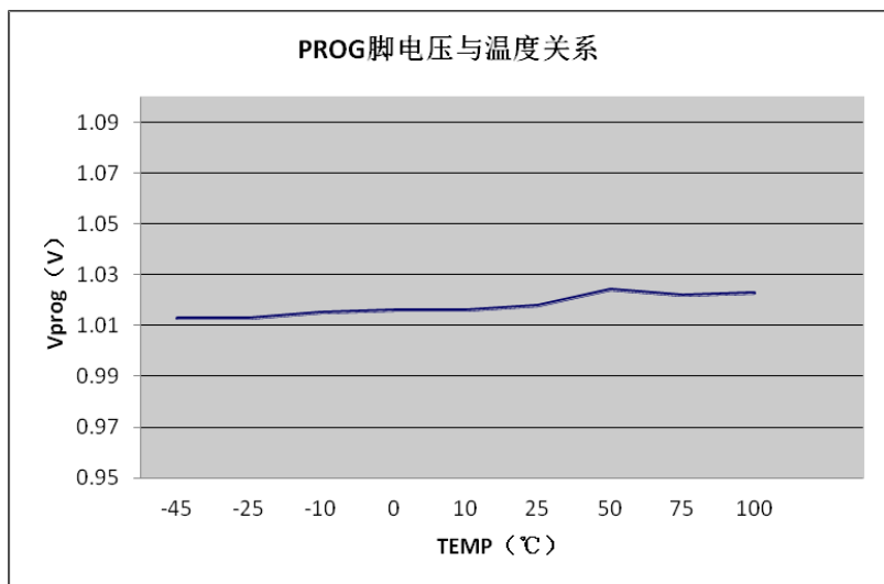
△Figure 11. PROG 脚电压温度曲线 (测试条件: VCC=5V, VBAT=3.7V, RPROG=2.4K)
