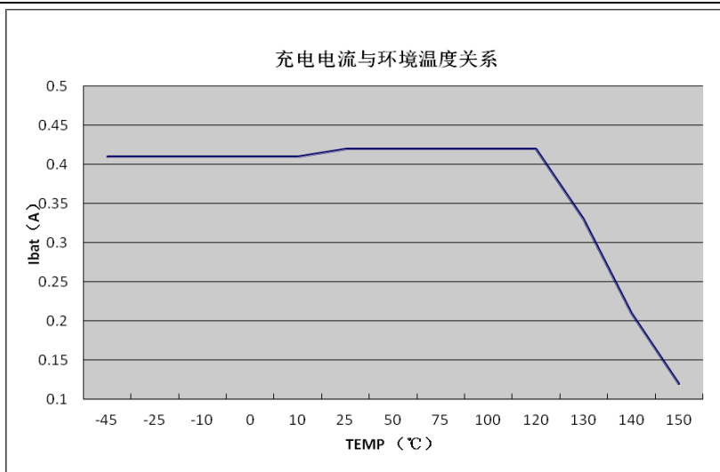
△Figure 13. 充电电流与环境温度关系 (VCC=5V, VBAT=4V, RPOG=3K)
