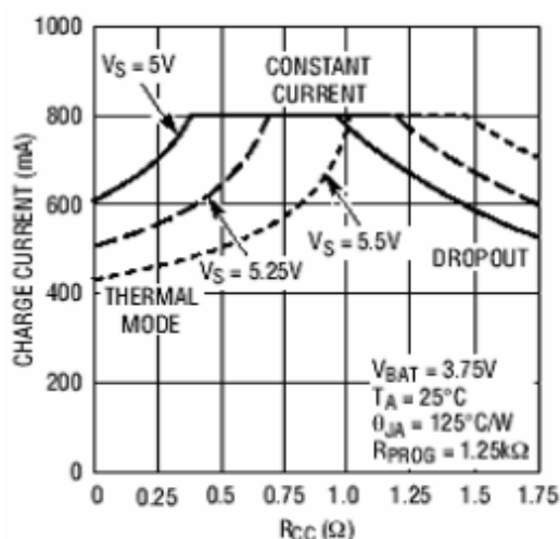
图 4 充电电流与 R_{\text{CC}} 的关系曲线
