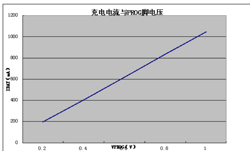
Figure 5. 充电电流与 PROG 脚电压（测试条件：VCC=5V，RPROG=1.2K）
