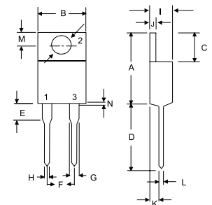
TO-220A
