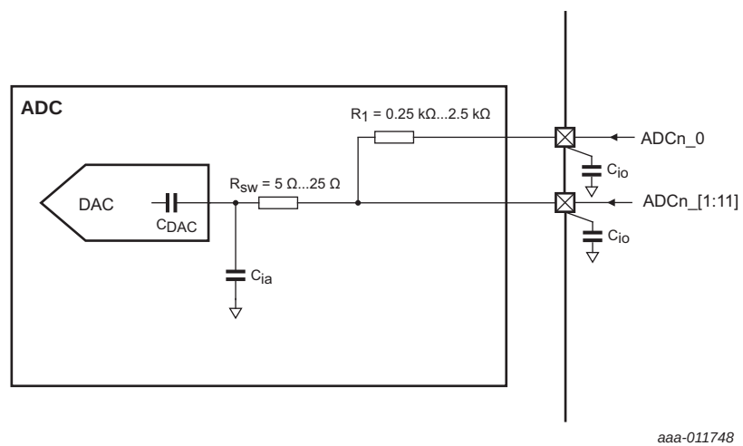
Fig 37. ADC input impedance
