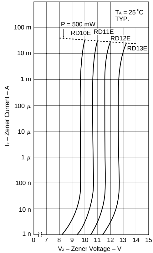
Fig. 4 ZENER CURRENT vs. ZENER VOLTAGE
