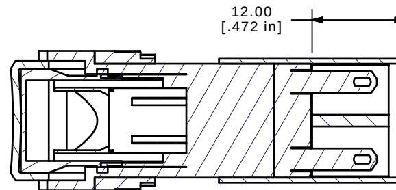
SECTION A-A SCALE 1.50 : 1
