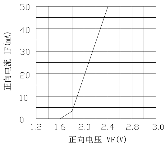
正向电流与正向电压
