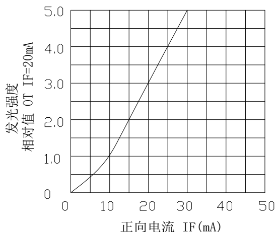
发光强度与正向电流
