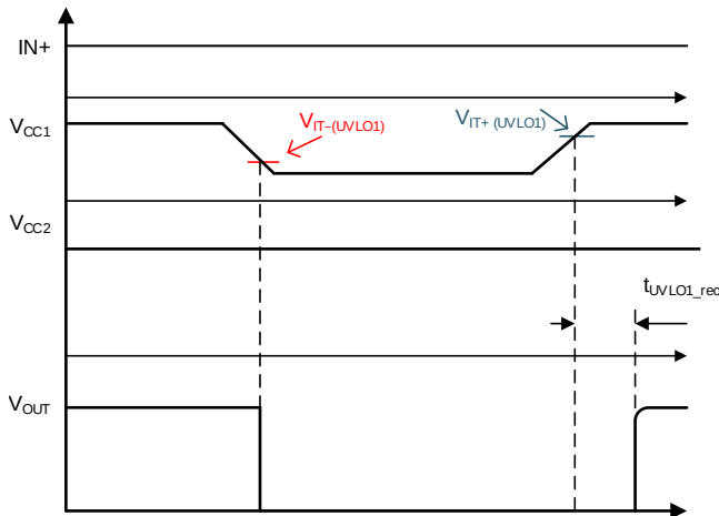
Figure 29. UVLO1 Functions
