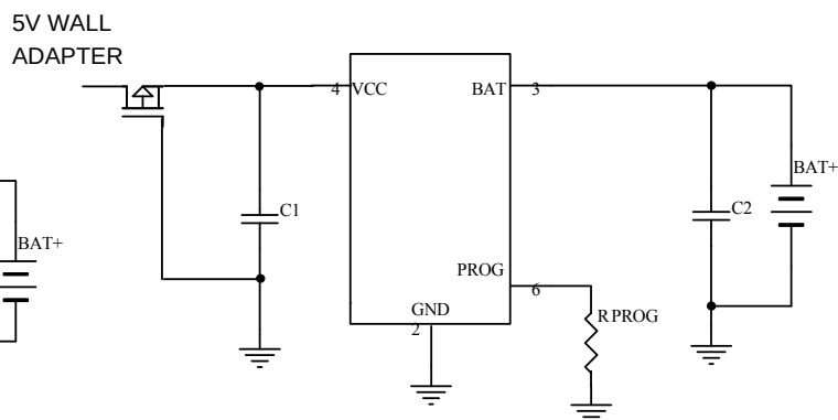
具有输入反向极性保护的充电器
