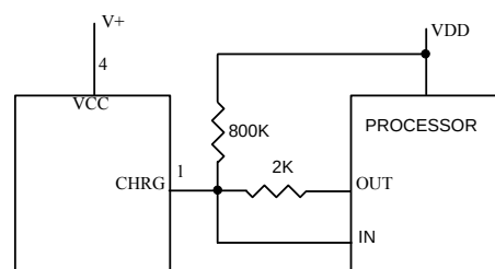
图 5：采用一个微处理器来确定 \overline{CHRG} 引脚状态
