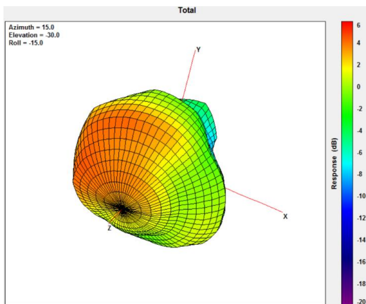
@2690MHz
