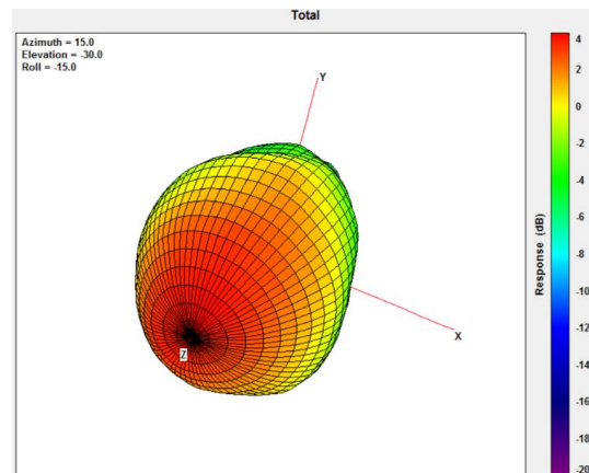
2170MHz
