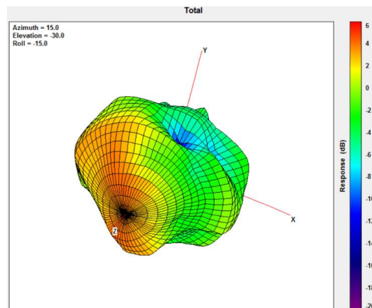
3500MHZ
