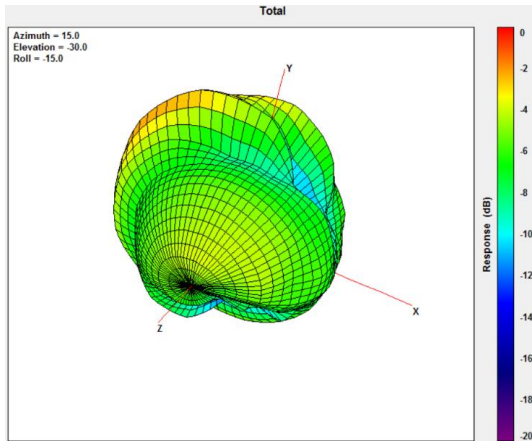
@704MHz
