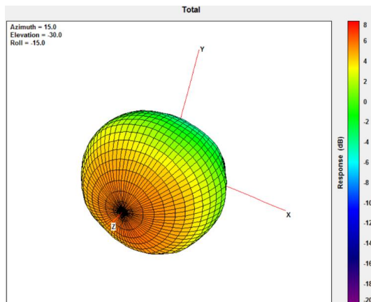
1710MHz
