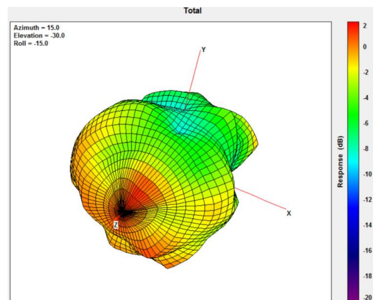
3500MHz
