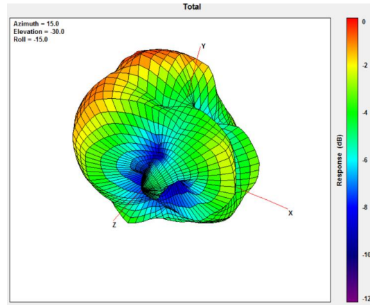
@960MHz
