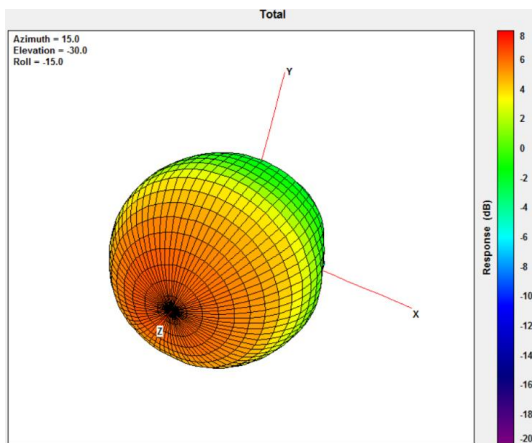
@1710MHz
