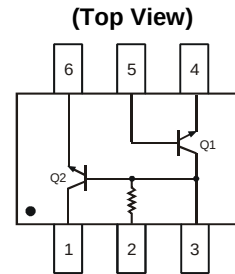
SOT26
