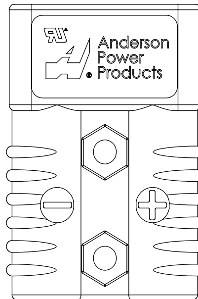
SB®175 - 2 Pole
