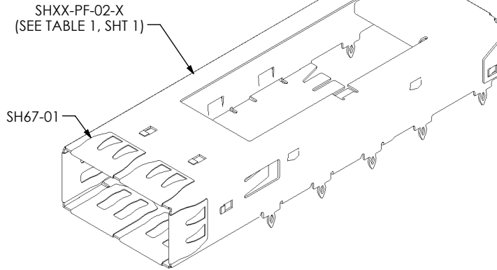
QSFP-PF-03
