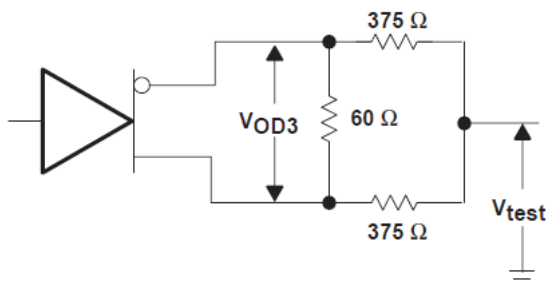
图 6-2. Driver V_{OD3}
