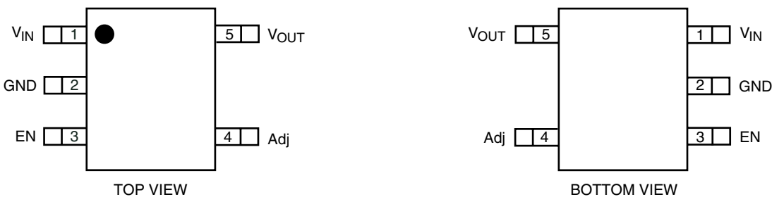
TSOT23-5L Package
