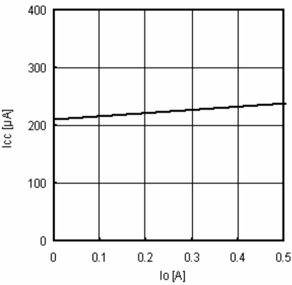
Fig.20 I_o - I_{cc}
