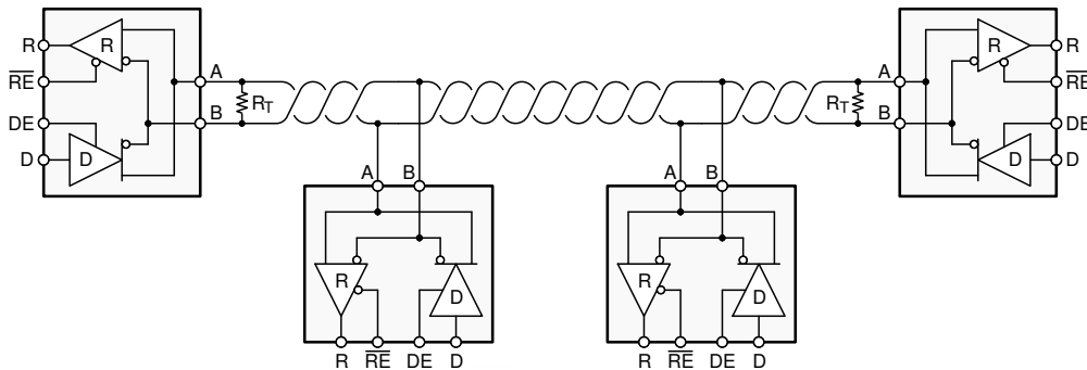
典型应用图
