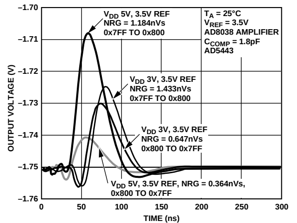
图29. 半量程转换, V_{REF} = 3.5\text{ V}
