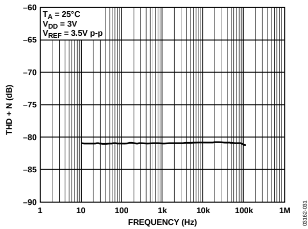
图31. THD和噪声与频率的关系
