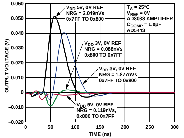
图28. 半量程转换, V_{REF} = 0\text{ V}
