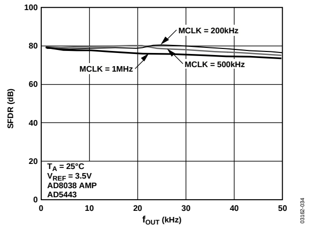
图33. 宽带SFDR与 f_{OUT} 频率的关系(AD5443)
