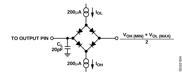
图 4. SDO时序规格的负载电路
