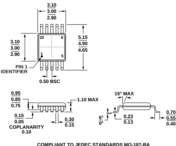
图51. 10引脚超小型封装[MSOP] (RM-10) 图示尺寸单位: mm
