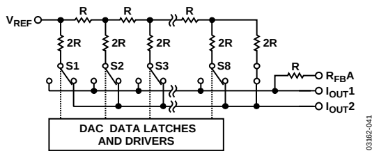
图40. 简化梯形图
