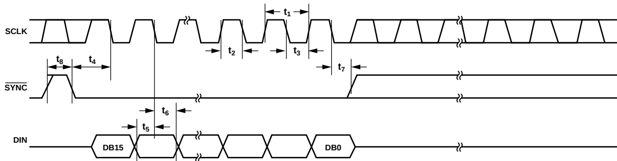
图2. 独立模式时序图
