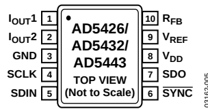
图5. 引脚配置
