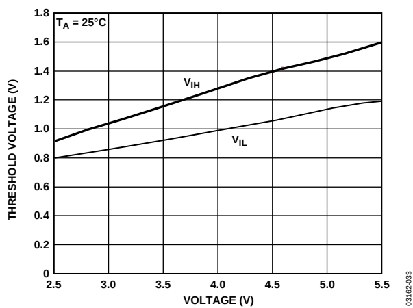
图32. 阈值电压与电源电压的关系
