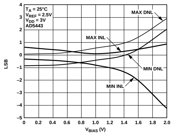
图16. 线性度与IOUT2上VBIAS电压的关系
