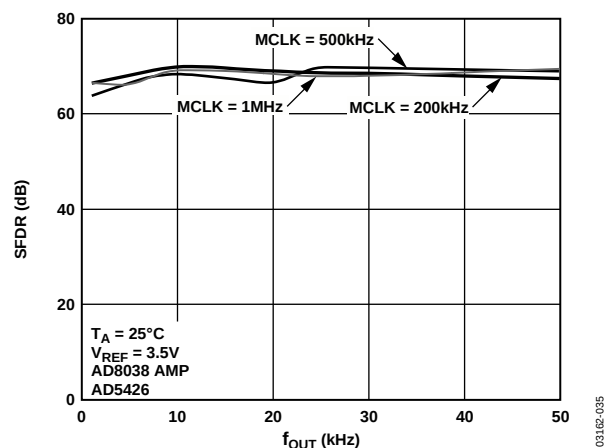
图34. 宽带SFDR与 f_{OUT} 频率的关系(AD5426)
