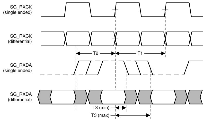
图 7-4. SGMII Timing
