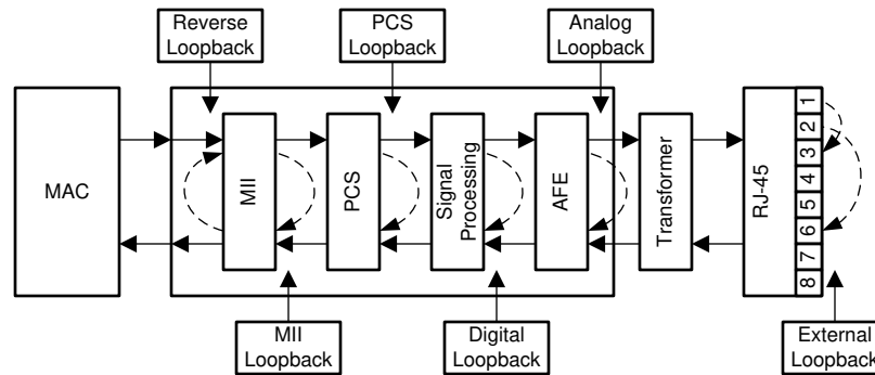
图 8-9. Loopbacks
