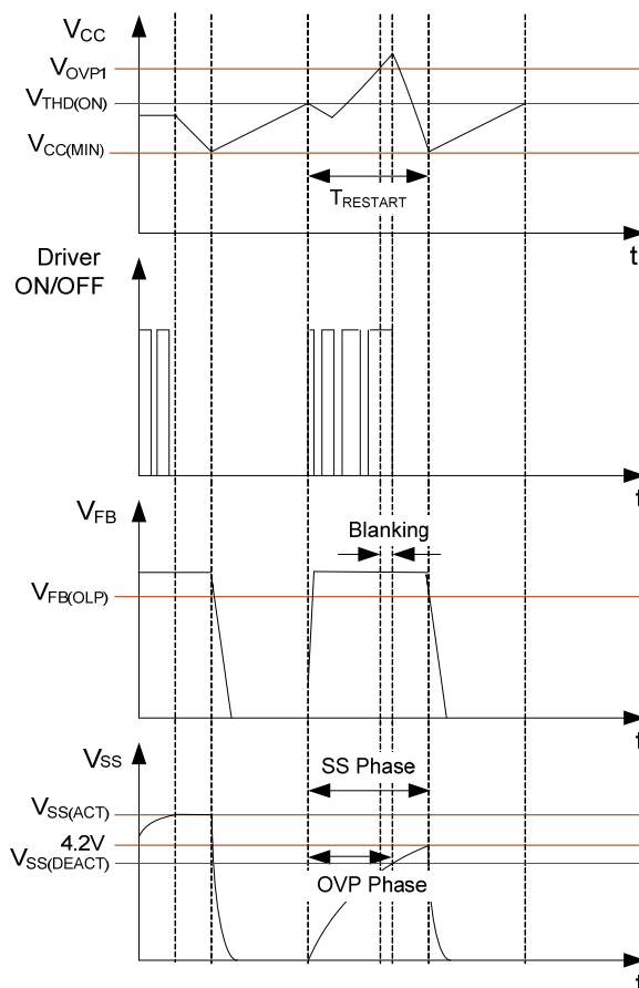
FIG.7 OVP case
