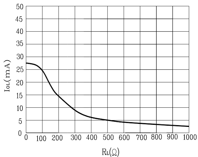
Fig. 4 I_{OL} - R_L
