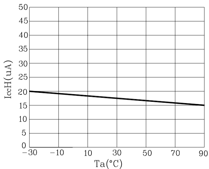
Fig. 3 I_{CCH} - T_a
