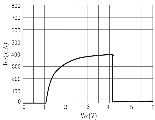
Fig. 2 I_{CC} - V_{CC}
