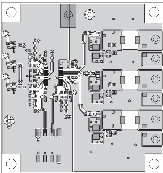
Top Side
